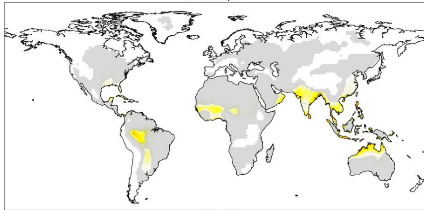
RCP 2.6
